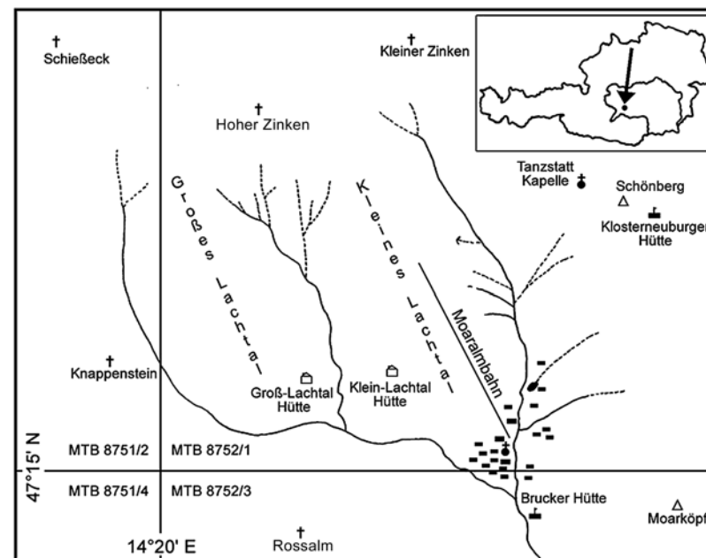
Abb. 1: Lage des Untersuchungsgebietes mit Grenzen der Grundfeldquadranten
