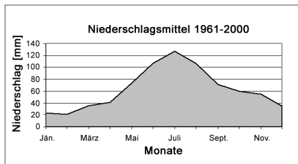
Abb. 2: Oberwölz - Langjährige Niederschlagsmittel (1961-2000)
